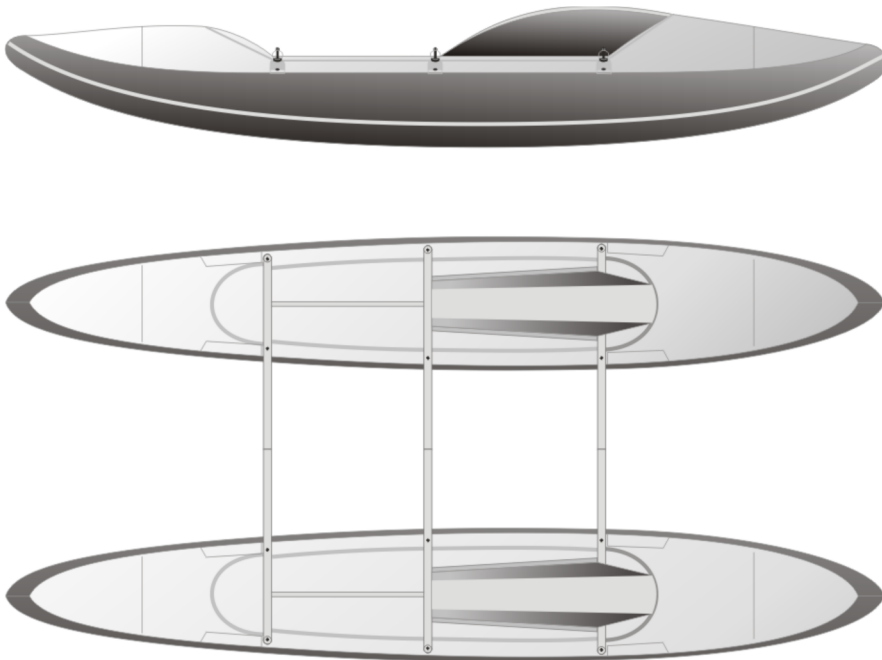
Внешний вид катамарана «КАСКАД-2».
